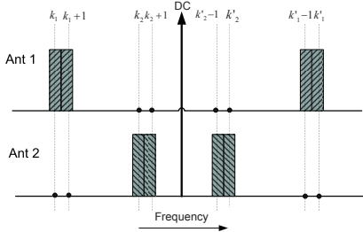
(b) SM-OFDM
