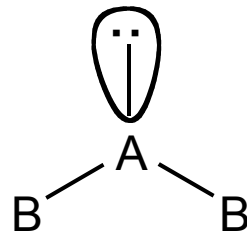
Bent
