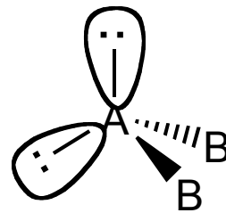
Bent
